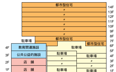
東西断面図
